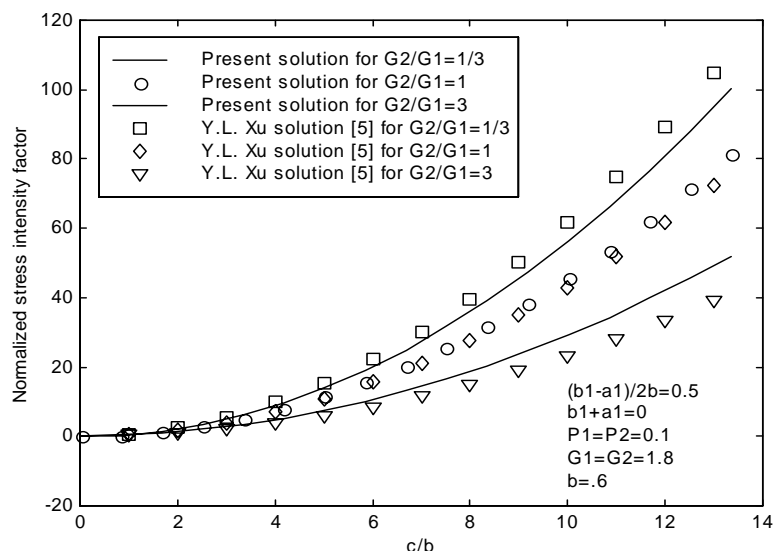
شکل ۱۱- ضریب شدت تنش بی بعد شده بر حسب پهنای حلقه برای کرنش صفحه‌ای
